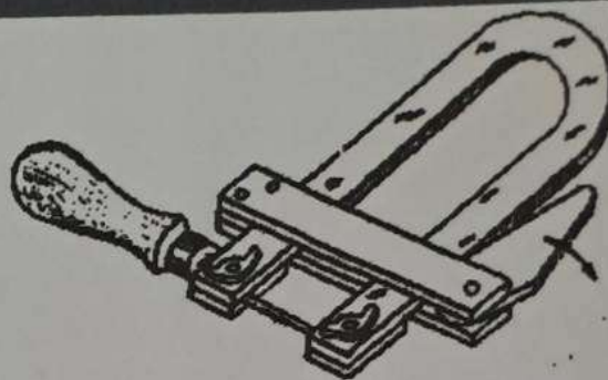
Рис. 7. Пристрій для натягування пилючки
